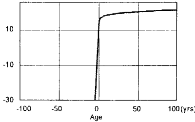
IV-4. Utility function
